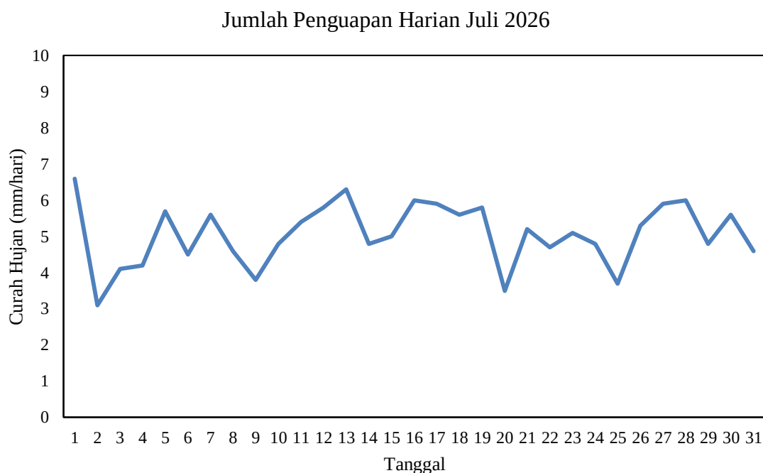
Gambar 2.8 Grafik Jumlah Penguapan Harian bulan Juli 2026 di Stasiun Meteorologi Mali - Alor
