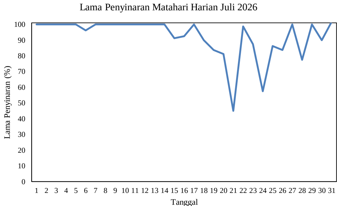
Gambar 2.7 Grafik Lama Penyinaran Matahari Harian bulan Juli 2026 di Stasiun Meteorologi Mali - Alor
