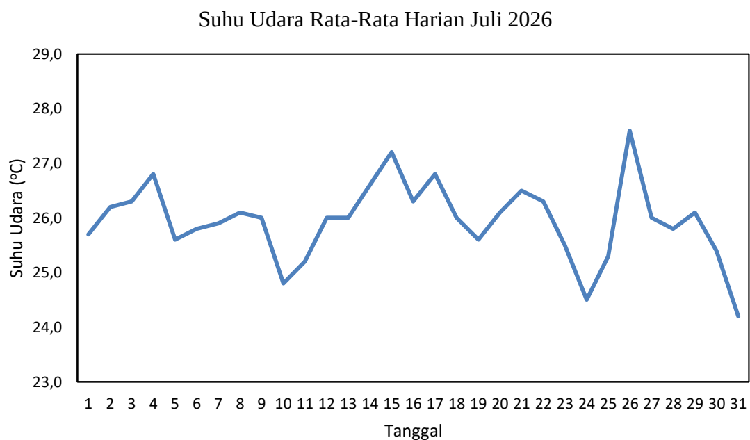
Gambar 2.1 Grafik Suhu Udara Rata-rata Harian Bulan Juli 2026 di Stasiun Meteorologi Mali - Alor
