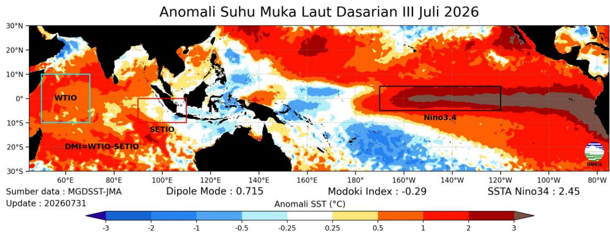
Gambar 3.2 Anomali Suhu Muka Laut di sekitar wilayah Indonesia pada Dasarian III bulan Juli 2026
