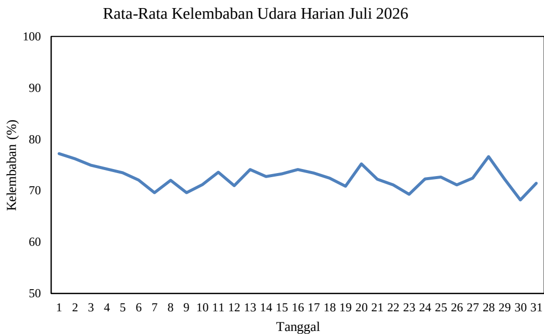
Gambar 2.5 Grafik Rata-rata Kelembaban Udara Harian Juli 2026 di Stasiun Meteorologi Mali - Alor
