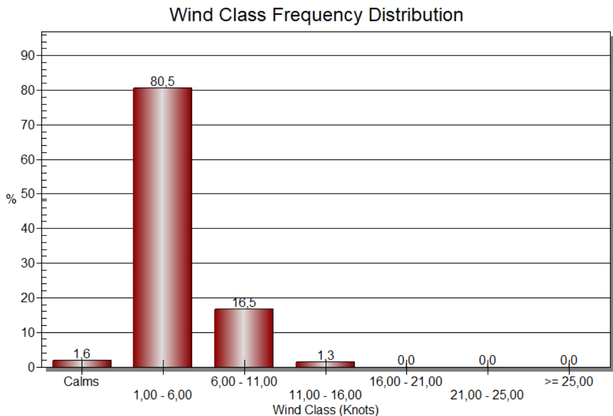
Gambar 2.10 Distribusi Frekuensi Angin Permukaan Bulan Juli 2026 di Stasiun Meteorologi Mali - Alor
