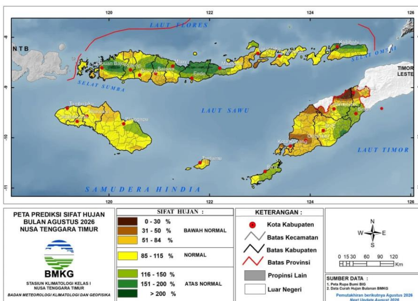
Gambar 4.2 Peta Prakiraan Sifat Hujan bulan Agustus 2026 wilayah provinsi Nusa Tenggara Timur
