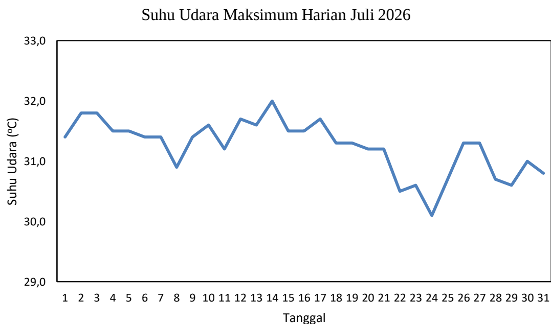
Gambar 2.2 Grafik Suhu Udara Maksimum Juli 2026 di Stasiun Meteorologi Mali - Alor
