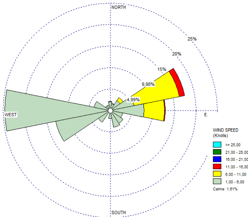
Gambar 2.9 Wind Rose Angin Permukaan Bulan Juli 2026 di Stasiun Meteorologi Mali - Alor
