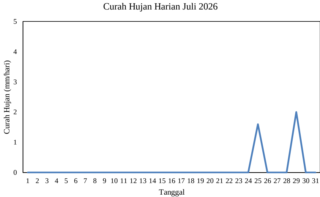
Gambar 2.4 Grafik Curah Hujan Harian Juli 2026 di Stasiun Meteorologi Mali - Alor
