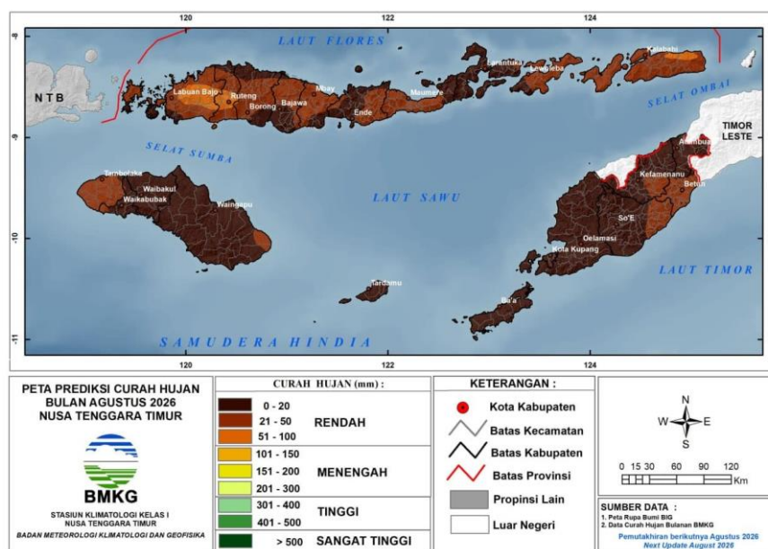
Gambar 4.1 Peta Prakiraan Curah Hujan bulan Agustus 2026 wilayah Provinsi Nusa Tenggara Timur
