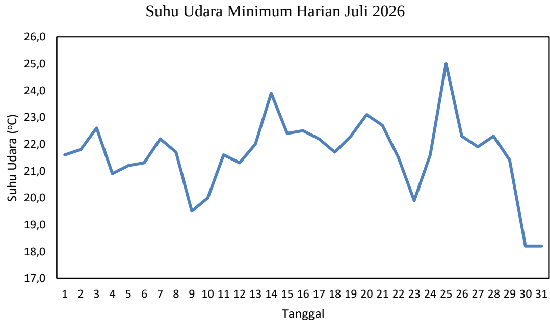
Gambar 2.3 Grafik Suhu Udara Minimum Juli 2026 di Stasiun Meteorologi Mali - Alor
