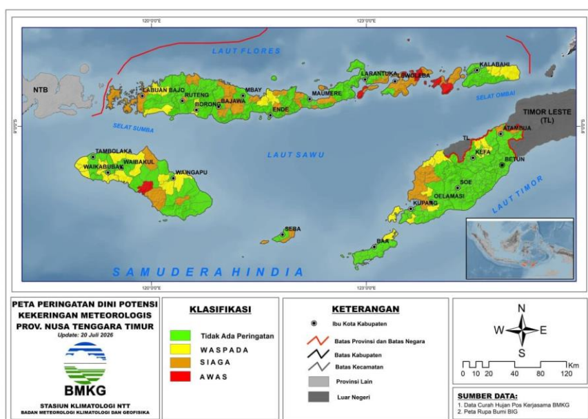
Gambar 4.4 Peta Peringatan Dini Potensi Kekeringan Meteorologis bulan Agustus 2026 wilayah provinsi Nusa Tenggara Timur
