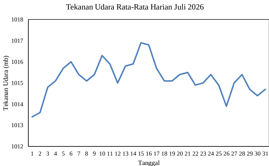
Gambar 2.6 Grafik Tekanan Udara Rata-rata Harian bulan Juli 2026 di Stasiun Meteorologi Mali - Alor
